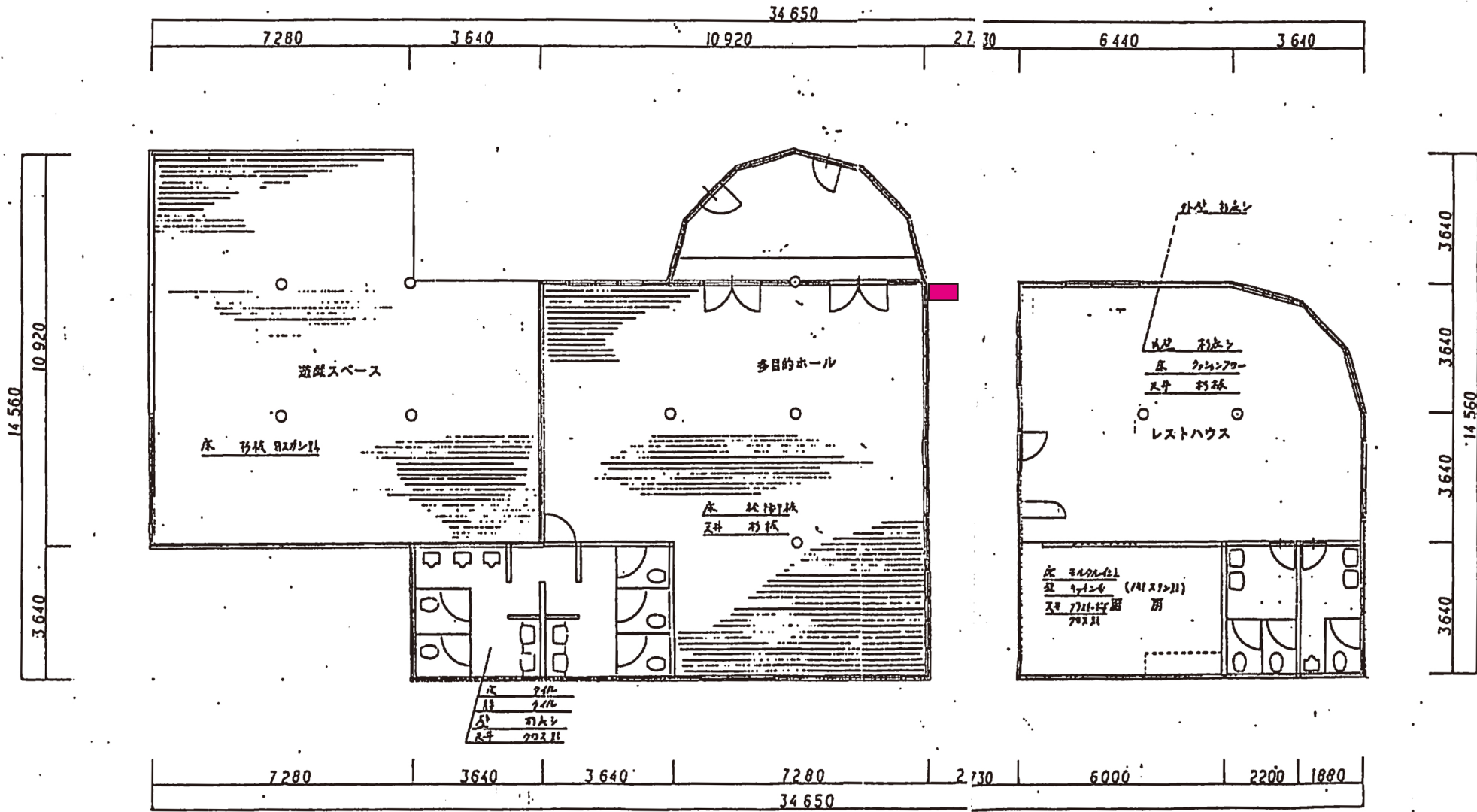
平面図 S=1/100
